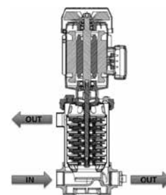
Versión R / conexiones roscadas 2 opciones (cambiando posición tapón): - en línea - entrada inferior y salida superior
