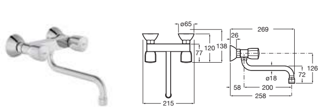
Brava Grifería mural para cocina o lavadero Con caño inferior giratorio y aireador Cromado A5A768EC00 € 107,00
