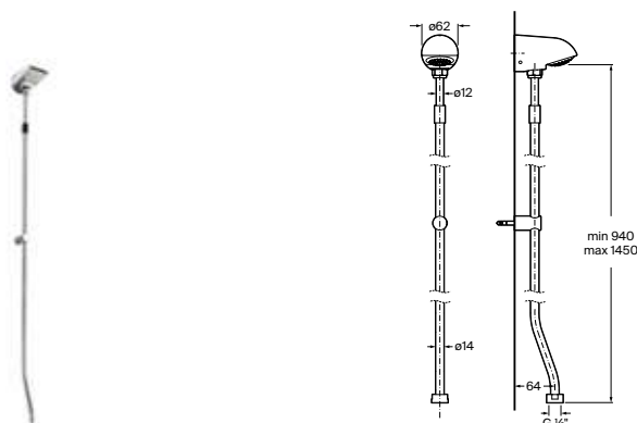
Conjunto de tubo, brida y rociador
