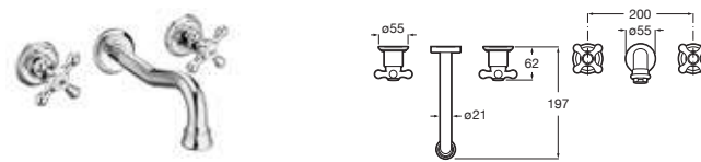
Grifería empotrable para lavabo Cromado A5A474BC00 € 243,00
