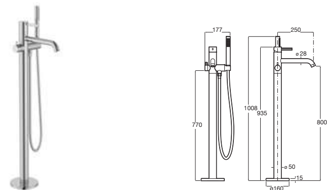
Grifería monomando de pie para baño-ducha Con inversor automático, ducha de mano, flexible de 1,5m, soporte articulado y columnas verticales de alimentación. A completar con Box instalación
