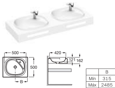
Compatibilidad de cubetas según ancho de encimera
