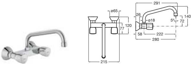
Brava Grifería mural para cocina Con caño superior giratorio y aireador Cromado A5A748EC00 € 107,00
