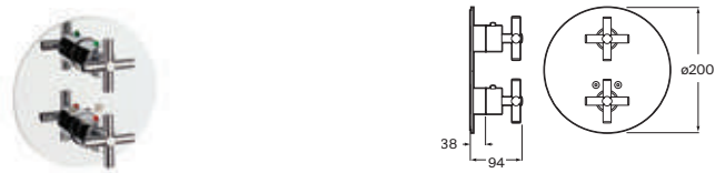
Grifería termostática empotrable para baño- ducha Con desviador-regulador de caudal Cromado A5A0643C00 € 796,00 Según tipo de instalación deberá colocarse una llave de paso
