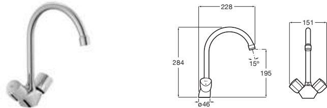
Brava Grifería para cocina y lavadero Con caño giratorio y aireador Cromado A5A848EC00 € 99,30
