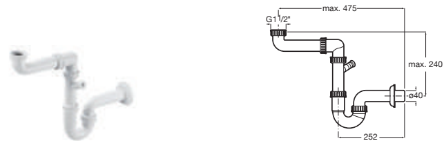
Sifón salvaespacio Blanco Para una cubeta A506405607 € 10,30
