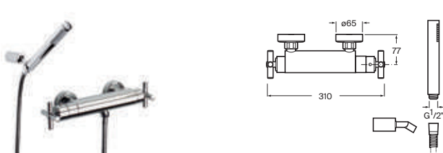
Grifería termostática exterior para ducha Con ducha de mano, flexible de 1,50 m y soporte articulado Cromado A5A1343C00 € 529,00
