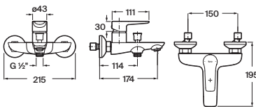
Grifería exterior para baño-ducha Con inversor automático con retención, ducha de mano Natura 80/1, flexible PVC de 1,7 m y soporte articulado
