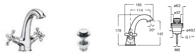
Grifería para lavabo con cuerpo liso Con aireador, desagüe click-clack y enlaces de alimentación flexibles Cromado A5A3A4BC00 € 183,00
