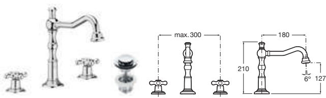
Grifería para lavabo con cuerpo liso Con caño central giratorio, aireador, desagüe click-clack y enlaces alimentación flexibles Cromado A5A444BC00 € 239,00
