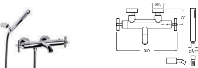
Grifería termostática exterior para baño- ducha Con inversor automático, ducha de mano, flexible de 1,70 m y soporte articulado Cromado A5A1143C00 € 767,00
