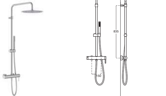
Columna para ducha monomando Con altura regulable y brazo de ducha orientable
