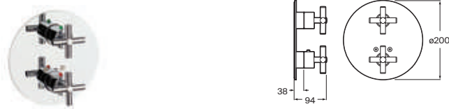
Grifería termostática empotrable para ducha Cromado A5A0743C00 € 772,00 Según tipo de instalación deberá colocarse una llave de paso
