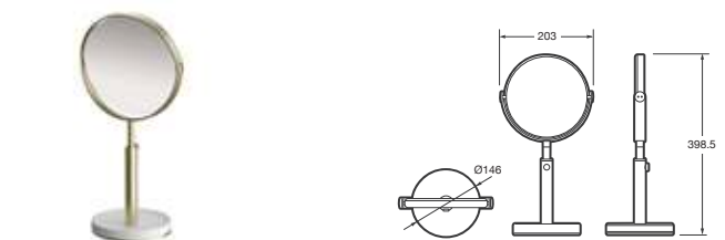
Espejo de aumento x5 con perfilera en acabado Greige y base en Off-White
