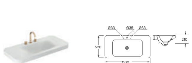
Lavabo de encimera en Surfex® con orificios para grifería
