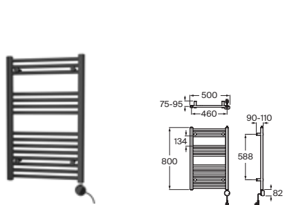
Toallero eléctrico 300 W Cromado A816640C00 € 365,00 Negro mate A816640NB0 € 247,00 Blanco brillo A816640P30 € 223,00
