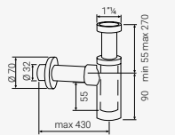
Sifón mural de sección redonda (latón)
