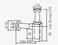
Sifón mural de sección cuadrada (latón)
