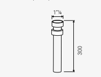
Prolongador para sifón plástico Blanco (De uso habitual el lavabos de altura como algunos Spot)
