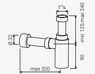
Sifón mural de sección redonda cromo (latón)
