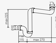
Sifón ahorro de espacio plástico Blanco (De uso habitual en la serie Program cuando se incorpora un estante bajo encimera)
