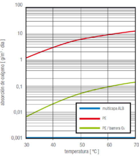
Curva de permeabilidad al oxígeno
