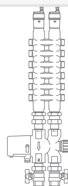
Tipo E Cómo tipo C pero válvula de zona serie 561T, 560T, 571T
