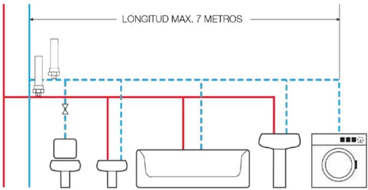
GRUPO DE BAÑO completo con WC a paso rápido = 8 unidades de carga 1 15M2 o WAM 1/2"
