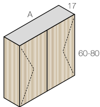
ARMARIO RANDA 1+1 PUERTAS Uñero Inferior.
