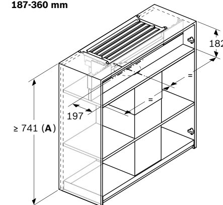
Montaje de la campana decorativa integrada con juego de recirculación de aire y prolongación de chimenea, 187-360 mm
