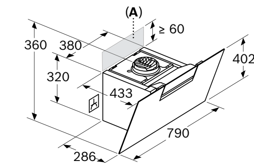
Aparato en recirculación sin conducto
