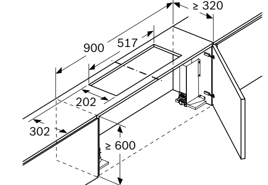
Montaje de la campana telescópica con juego de recirculación de aire
