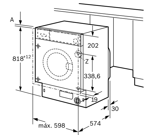
Detalle Z
