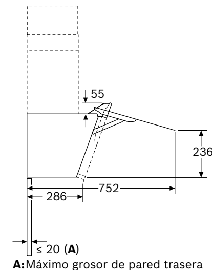
Aparato en recirculación sin conducto
