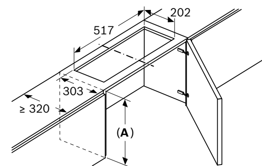
Montaje de la campana decorativa integrada con juego de recirculación de aire
