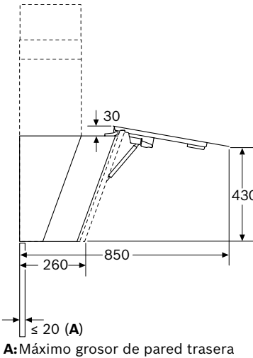
Aparato en recirculación sin conducto
