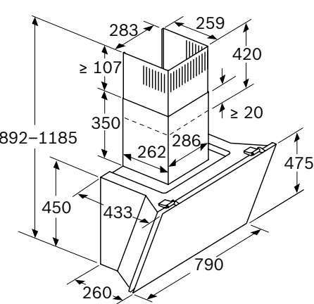
Aparato en recirculación
