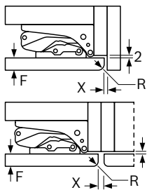
Dimensiones del espacio recomendadas para instalación de puerta fija
