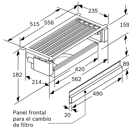
Montaje de la campana telescópica con juego de recirculación de aire y accesorio para ocultar el frente
