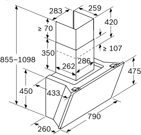
Aparato en salida de aire al exterior
