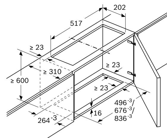
Montaje del módulo de integración con juego de recirculación de aire
