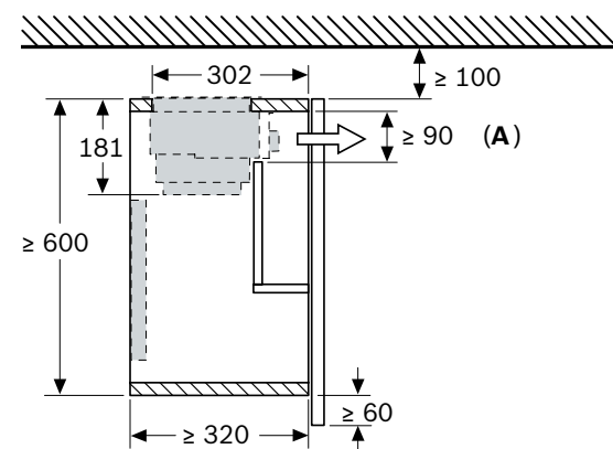
Montaje de la campana telescópica con juego de recirculación de aire y accesorio para ocultar el frente
