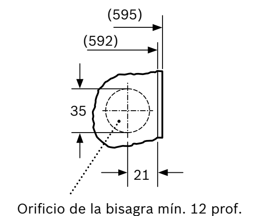
Detalle Z
