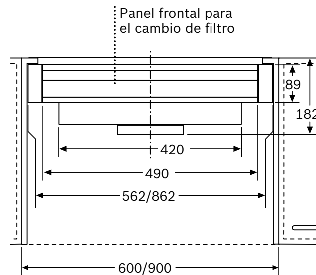
Montaje de la campana decorativa integrada con juego de recirculación de aire
