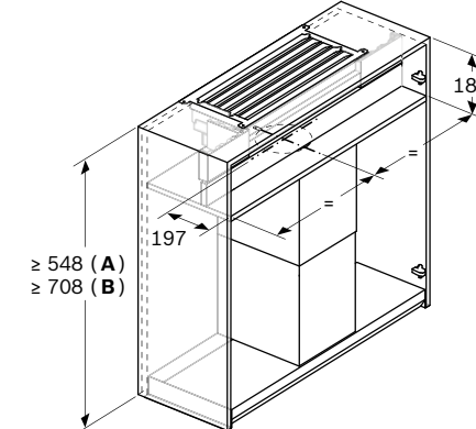
Montaje de la campana decorativa integrada con juego de recirculación de aire y prolongación de chimenea
