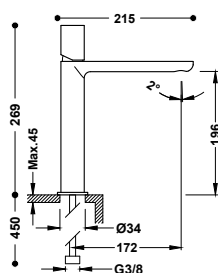
Latiguillos de alimentación flexibles G3/8.
