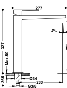
Latiguillos de alimentación flexibles G3/8.
