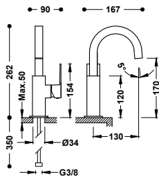
Grifo monomando con maneta lateral para lavabo Latiguillos de alimentación flexibles G3/8.
