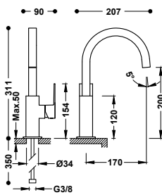
Grifo monomando alto con maneta lateral para lavabo Latiguillos de alimentación flexibles G3/8.
