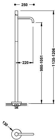
Grifo monomando con toma a suelo para lavabo Caja empotrada (Ref. 26285350) no incluida. 1 columna vertical de alimentación de agua a suelo.
