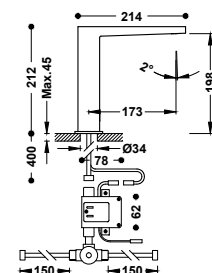
Grifo electrónico con sistema premezclador para lavabo Accionado mediante sensor de infrarrojos. Incluye una válvula mezcladora de 2 aguas con tubos flexibles.
