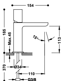
Latiguillos de alimentación flexibles G3/8.
