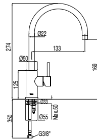
Grifo monomando con maneta lateral para lavabo Latiguillos de alimentación flexibles G3/8.
