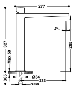
Grifo monomando XXL para lavabo Latiguillos de alimentación flexibles G3/8.
