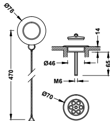
Cazoleta plana de desagüe con kit de enganche de cadenilla y tapón para bañera Cadenilla: 450 mm. Cazoleta: Ø 70 mm. Tapón metálico.
