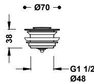
Válvula de desagüe Click-clack con tapón oculto para bañera Función Click-clack. Tapón: Ø 36 mm.
