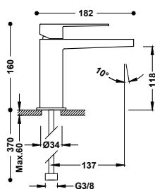
Latiguillos de alimentación flexibles G3/8.
