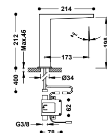
Grifo electrónico de 1 agua para lavabo Accionado mediante sensor de infrarrojos.
