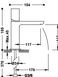
Caño cerrado con salida del agua en cascada. Latiguillos de alimentación flexibles G3/8. Se incluyen 2 llaves de regulación con filtro (ref: 9134525).
