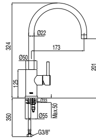
Grifo monomando alto con maneta lateral para lavabo Latiguillos de alimentación flexibles G3/8.
