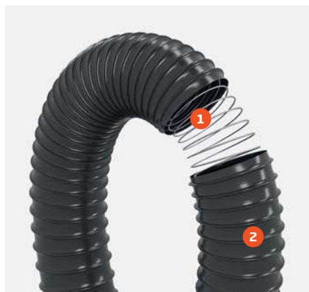
1. Espiral de acero cincado. 2. PVC plastificado.
