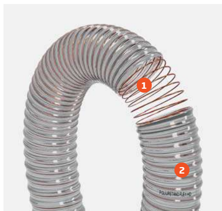
1. Espiral de acero cobreado. 2. Poliuretano transparente base poliéter.
