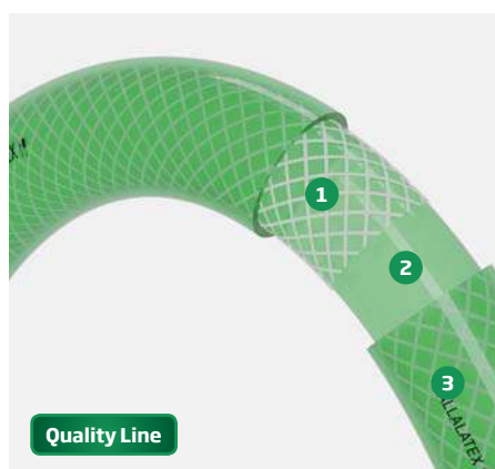
1. Capa intermedia: refuerzo de malla de hilo de poliéster. 2. Capa interior de material tacto látex de uso alimentario. 3. Capa exterior de material tacto látex de uso alimentario.
