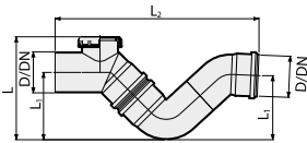
Sifón Colector en línea Macho/Hembra con registro
