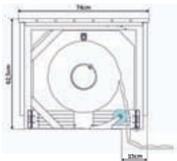
Dimensiones exteriores
