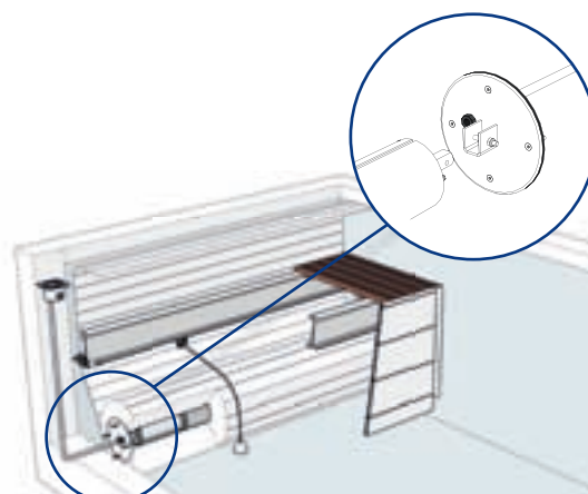
Playa sumergida motor en el eje fijación pared mediante pletinas
