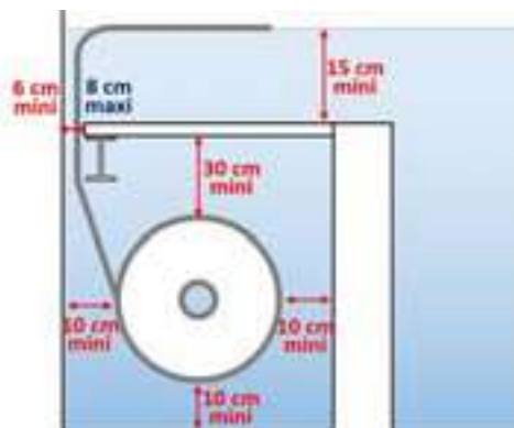
Cotas mínimas a respetar Cubiertas Playa Sumergida
