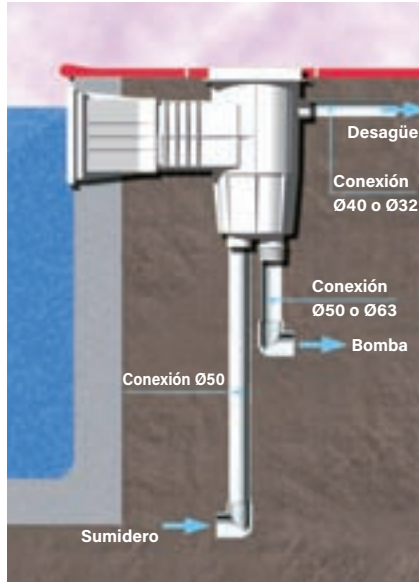
Instalación boquillas
