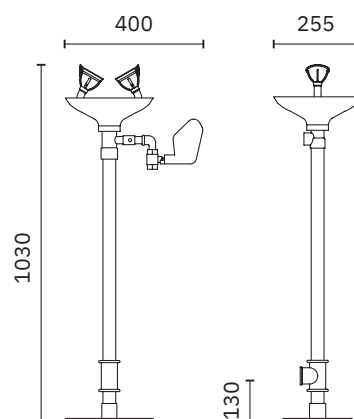
Lavajos de emergencia con pedestal
