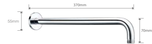
Ref.: BPR001 Tubo a pared redondo. Latón acabado cromo.
