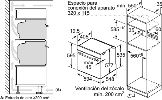
Instalar dos aparatos uno encima de otro Circulación de aire
