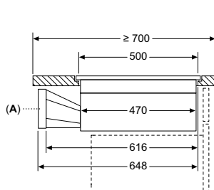
Placas flexInducción y combiInducción con extractor integrado
