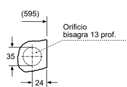
Detalle Z
