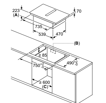
Placas flexInducción EX875LX67E, EX851HJ26E y combiInducción ED851HQ26E de 80 cm con extractor integrado en mueble de 60 cm
