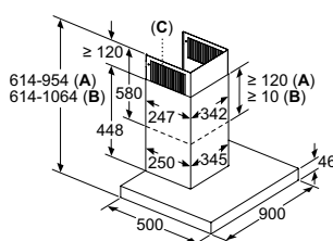
A: Salida de aire al exterior B: Circulación de aire C: Salida de aire: montar con las ranuras de la salida de aire al exterior hacia abajo
