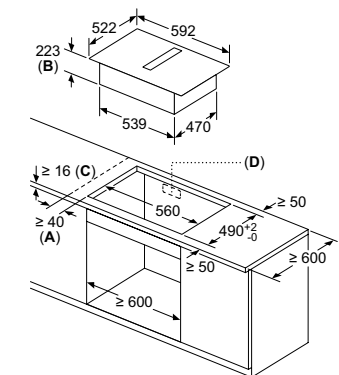
Placa combiInducción ED631HQ26E de 60 cm con extractor integrado
