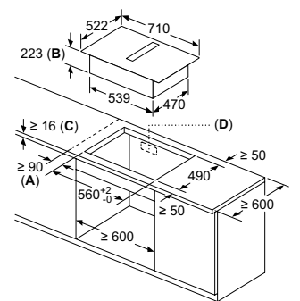
Placa combiInducción ED751HQ26E de 70 cm con extractor integrado
