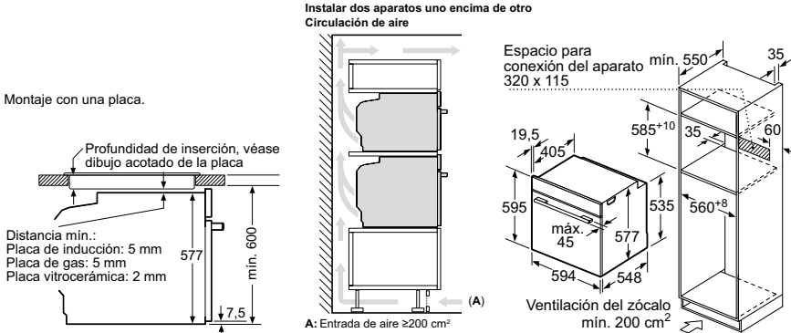
Instalar dos aparatos uno encima de otro Circulación de aire
