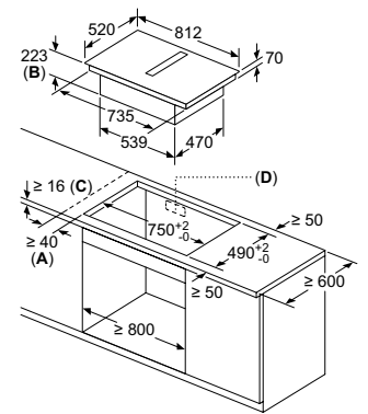
Placa flexInducción EX875LX67E de 80 cm con extractor integrado en mueble de 80 cm
