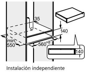
Instalación independiente
