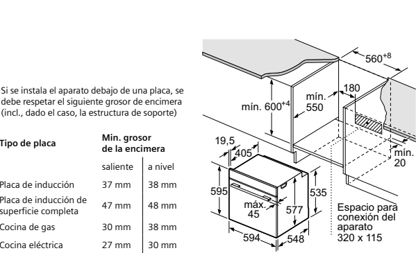
Montaje con una placa.
