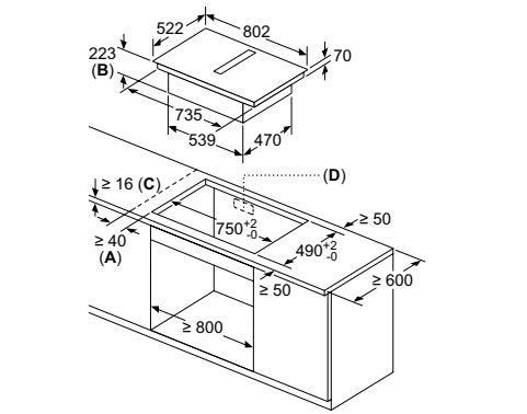
Placa flexInducción EX851HJ26E y combiInducción ED851HQ26E de 80 cm con extractor integrado en mueble de 80 cm
