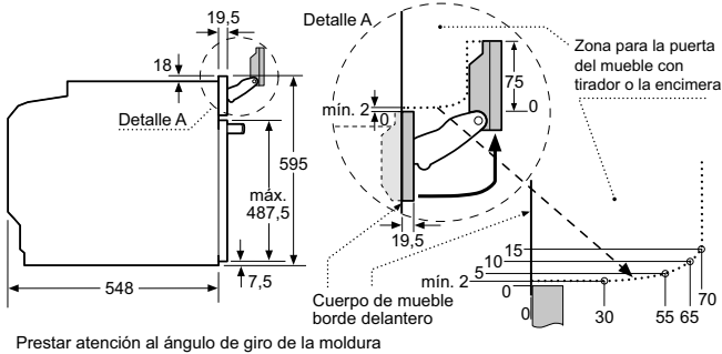
Prestar atención al ángulo de giro de la moldura
