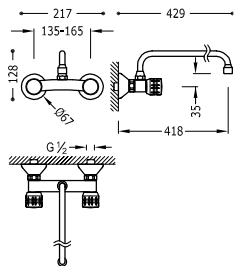
Grifo bimando mural para cocina Con caño superior. Distancia a pared: 418 mm.
