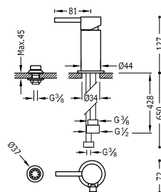
Grifo monomando para bidé con transferencia a duchita Con inversor para duchita. Latiguillos de alimentación flexibles G3/8.
