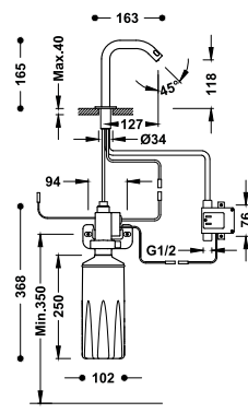
Grifo electrónico de 1 agua con dispensador de jabón automático para lavabo
