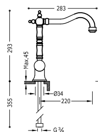
Grifo monomando para cocina Con latiguillos de alimentación flexibles G3/8.
