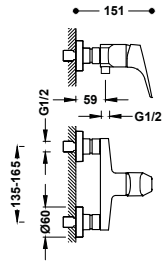
Grifo monomando mural para ducha Sin complementos.
