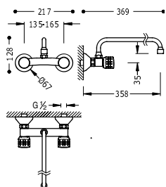
Grifo bimando mural para cocina Con caño superior. Distancia a pared: 358 mm.
