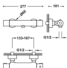
Grifo termostático mural para ducha Ducha de mano anticalcárea: Ø 100 mm. Soporte orientable para ducha de mano. Flexo metálico.
