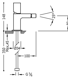
Grifo monomando para bidé Rótula orientable. Latiguillos de alimentación flexibles G3/8.
