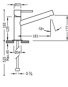
Grifo monomando para lavabo Caño largo. Latiguillos de alimentación flexibles G3/8.
