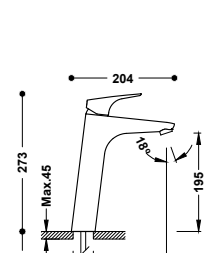
Grifo monomando alto para lavabo con Tres-Duo Latiguillos de alimentación flexibles G3/8.
