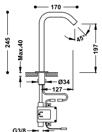
Grifo electrónico de 1 agua para lavabo Accionado mediante sensor de infrarrojos.
