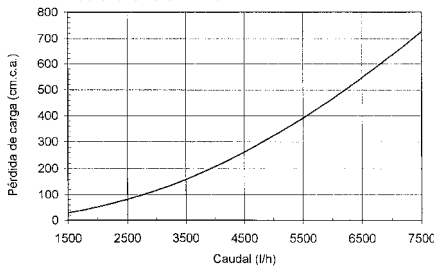
VÁLVULA DE 1"
