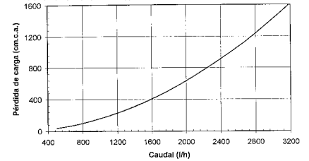
VÁLVULA DE 1/2"
