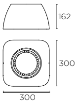
71-9995 - DC - DC
