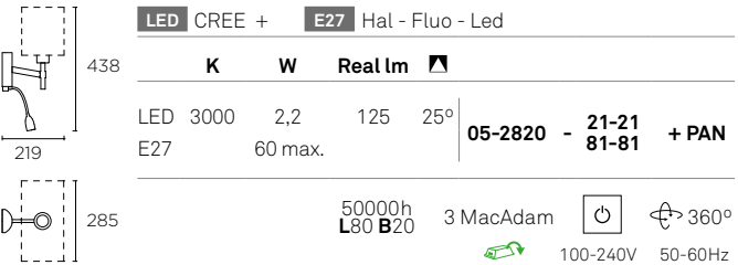
05-2820-21-21+PAN-176-14
