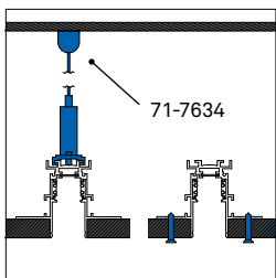
Instalación / Instalação
