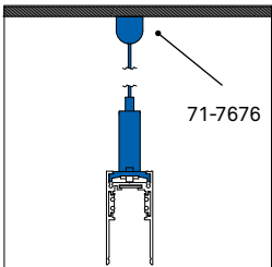
Instalación / Instalação
