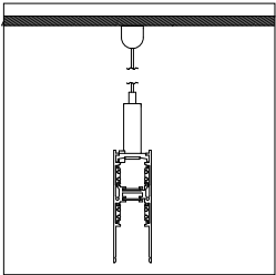
Instalación / Instalação
