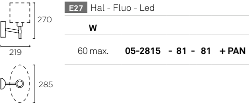
05-2815-81-81+PAN-177-BY
