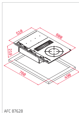
AFC 87628
