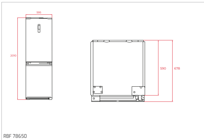
RBF 78650
