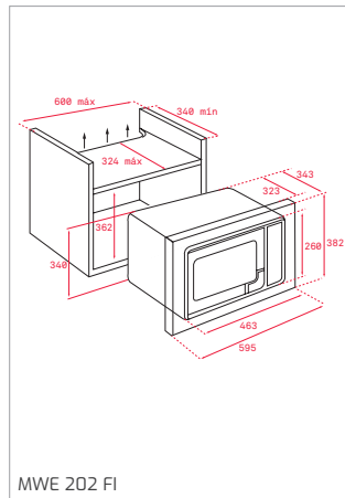
MWE 202 FI
