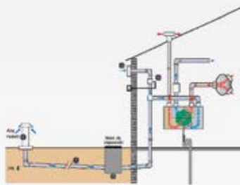
Registro en vivienda sin sótano
