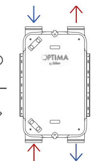
Modelo flujos de aire versión derecha Ref: DFOPTIMA2BPR
