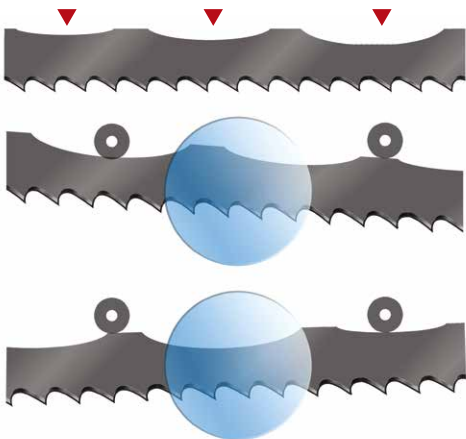
Imagen exagerada de la sierra con tecnología SPARC®
