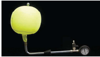
BALONES OBTURADORES PARA PE
