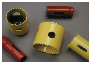
FRESA DE PASO VARIABLE PARA TUBERÍAS RÍGIDAS
