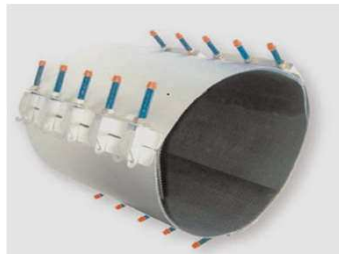
ABRAZADERA DE REPARACION TS30 - 3 SECTORES
