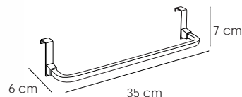
50101 Barra colgar Hang bar Rail accro chant
