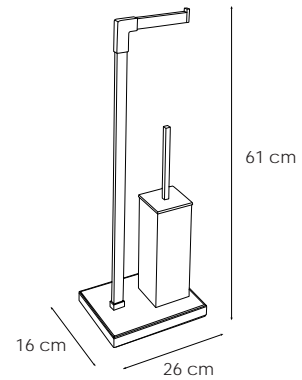
40241 Portaescobillero 041 Brush holder 041 Porte-brosse pied 041
