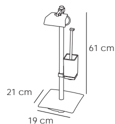
40223 Portaescobillero 023 Brush holder 023 Porte-brosse pied 023
