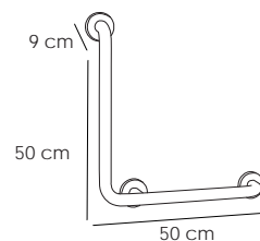
10809 Ayuda-09 Asa angular Inox Satin 100 € Help-09 Angular handle Aide-09 Anse angulaire
