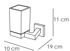
11708 Portavasos Cromo 39 € Glass holder Porte-verre
