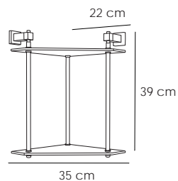
10142 Rinconera Deco 3 Lejas Cromo 160 € Three far corner shelf Deco Etagère d'angle Deco trois loi
