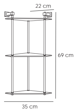
10142 Rinconera Deco 3 Lejas Cromo 160 € Three far corner shelf Deco Etagère d'angle Deco trois loi
